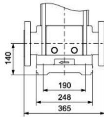
DIN FLANGE(SMVR)/F
