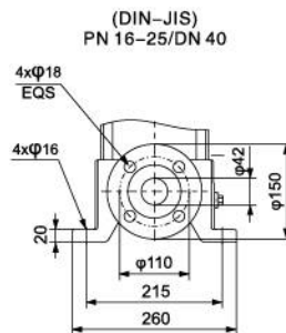
DIN FLANGE(SMVR)/F
