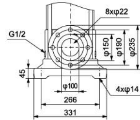
PN 25-40/DN 100
