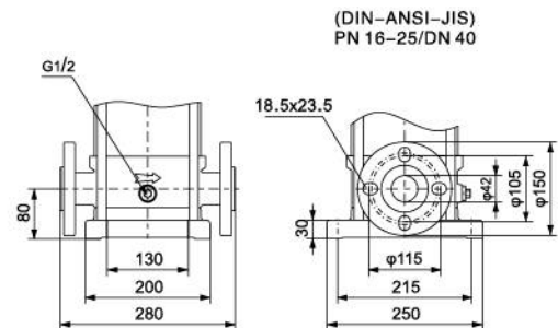
DIN FLANGE(SMVS)/F
