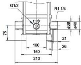
CLAMP CONNECTOR(SMVS)/K
