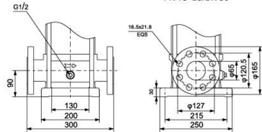
DIN FLANGE(SMVS)/F
