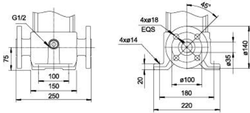
DIN FLANGE(SMVR)/F
