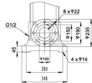
PN 25-40/DN 100
