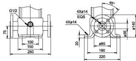
DIN FLANGE(SMVR)/F
