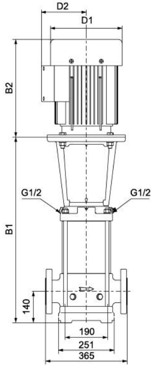
DIN FLANGE(SMVS)/F
