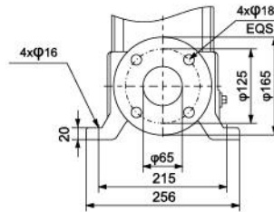
DIN FLANGE(SMVR)/F
