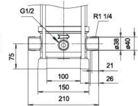
CLAMP CONNECTOR(SMVS)/K
