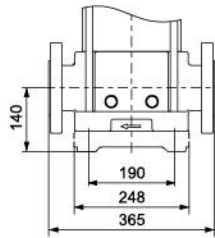
DIN FLANGE(SMVR)/F
