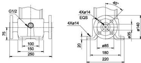
DIN FLANGE(SMVR)/F
