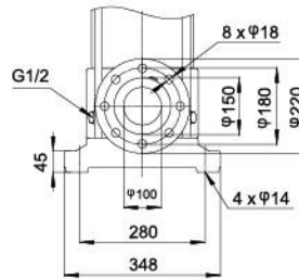
PN 16/DN 100
