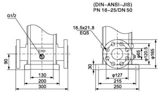
DIN FLANGE(SMVS)/F
