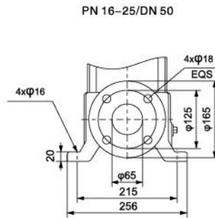
DIN FLANGE(SMVR)/F
