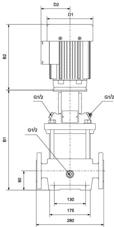
DIN FLANGE(SMVR)/F
