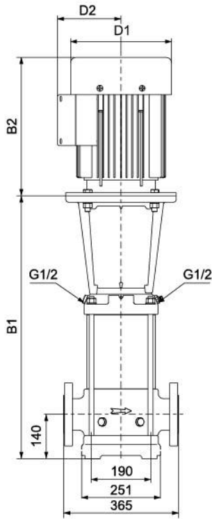
DIN FLANGE(SMVS)/F
